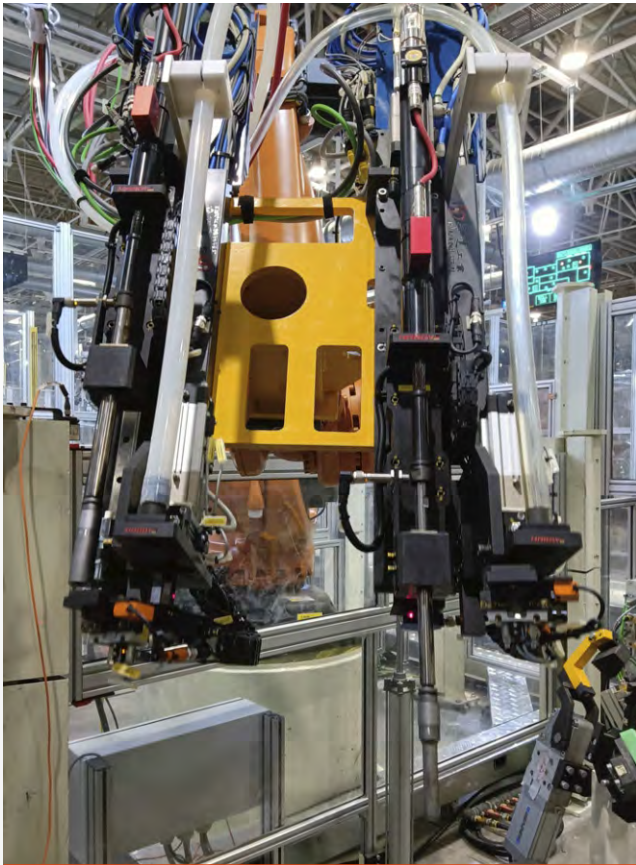
后盖铰链螺栓及球头螺栓自动送钉装配系统
