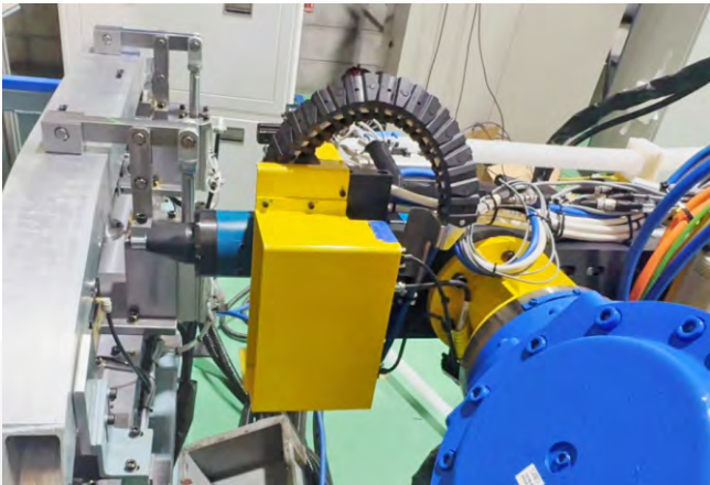
前保铆螺母自动铆接
