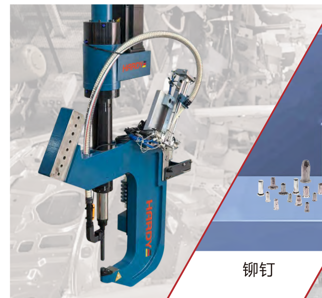
铆接装备
